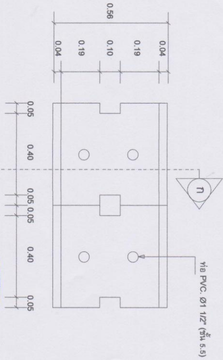
แบบแปลนรางระบายน้ำ
